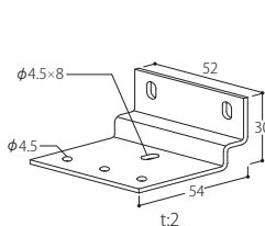
フレーム取付金具
