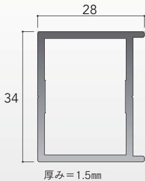
【メインフレーム】 原寸大
