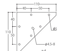
コーナー取付金具
